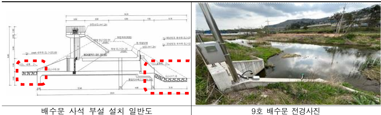
[그림 1] 배수문 하상보호공 설치 일반도 및 전경사진
